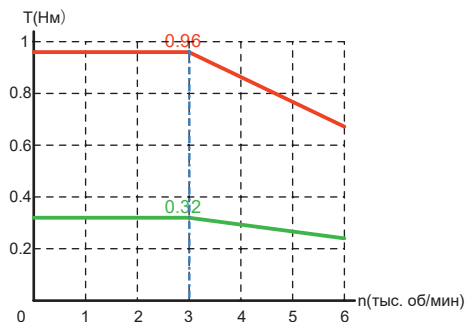
V7E-L04A-R6030-□□
