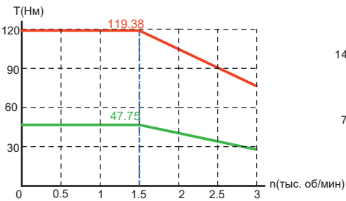
V7E-M1 8□-7R515-□□H
