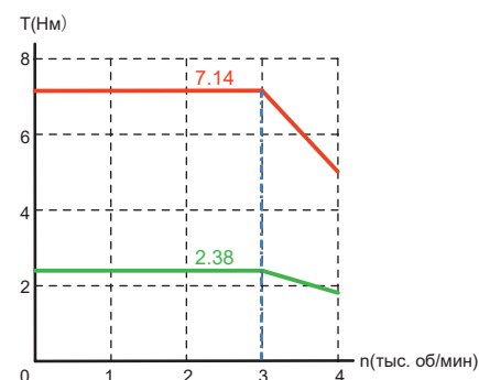
V7E-M11A-1R230-□□
