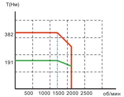
VM7-M20D-03015- □1FN
