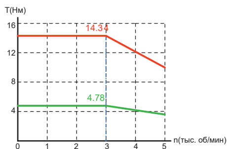
V7E-M11A-1R530-□□
