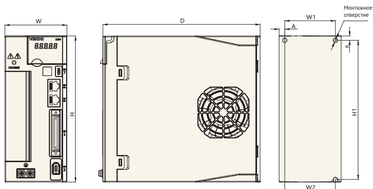
Типоразмер В
