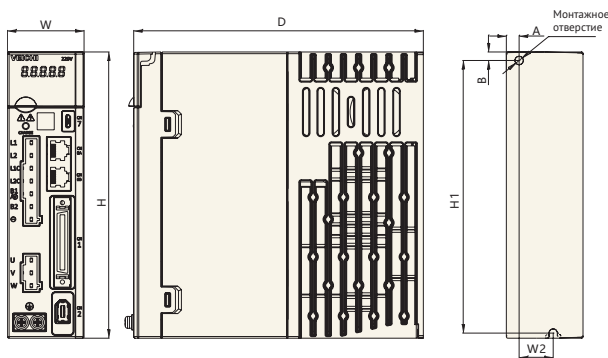
Типоразмер А
