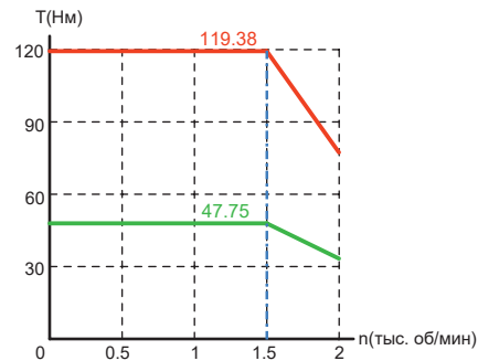
V7E-M18 □-7R515-□ □
