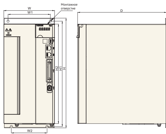
Типоразмер D
