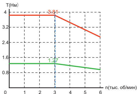
V7E-L08A-R7530-□□L
