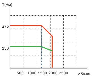
VM7-M20D-03715- □1FN
