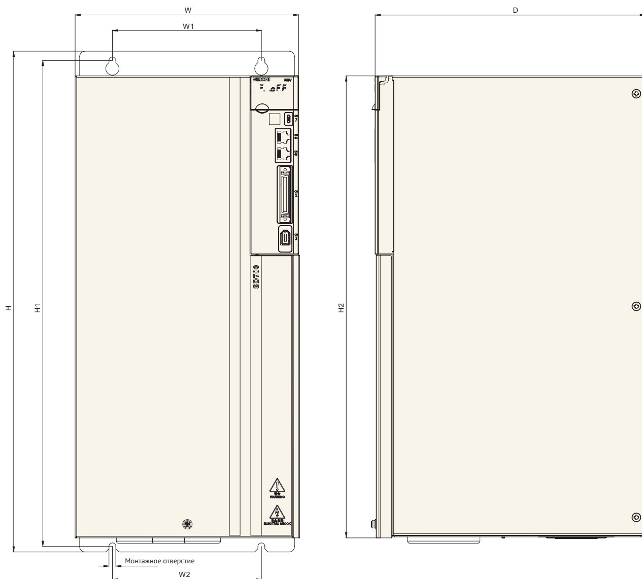
Типоразмер E/F
