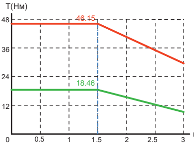
V7E-M1 8□-2R915-□□H
