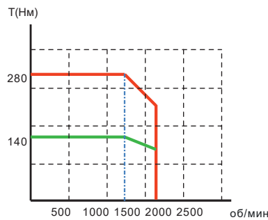
VM7-M20D-02215- □1FN
