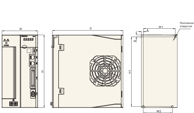
Типоразмер С
