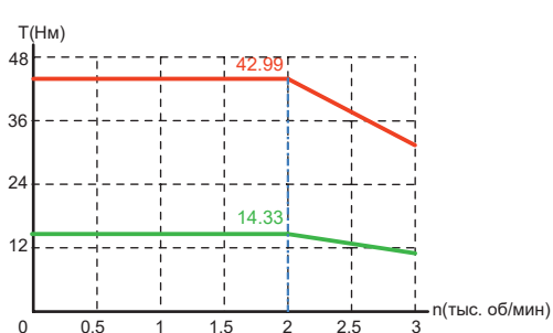
V7E-M13 □-3R020-□ □
