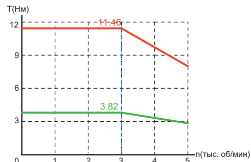
V7E-M11A-1R230-□□
