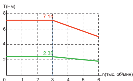
V7E-M11A-1R530-□□
