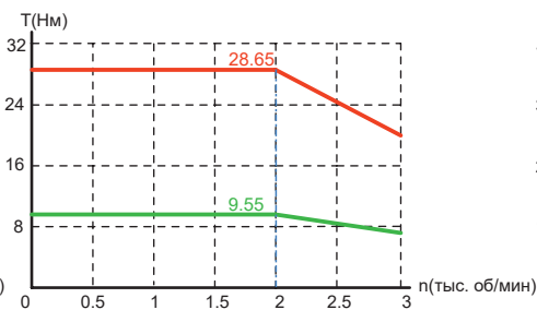
V7E-M13 □-2R020-□ □
