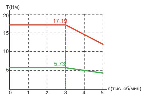
V7E-M11A-1R830-□□
