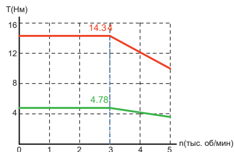
V7E-M11A-1R530-□□
