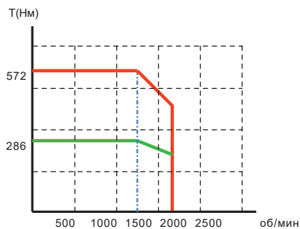
VM7-M20D-04515- □1FN
