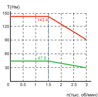
V9E-M18D-7R515
