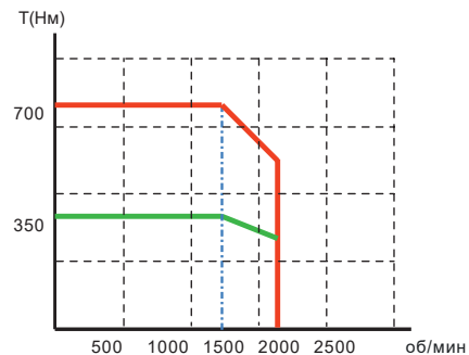
VM7-M20D-05515- □1FN
