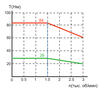
V9E-M18D-4R415
