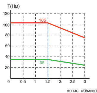
V9E-M18D-5R515
