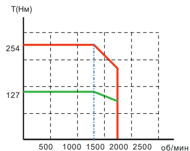
VM7-M20D-02015- □1FN
