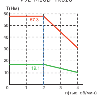
V9E-M18D-4R020
