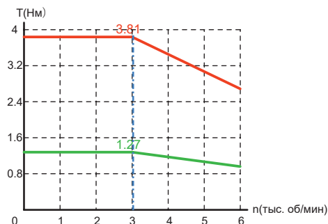
V7E-L08A-R7530-□□L
