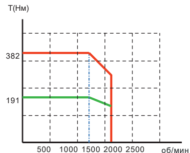
VM7-M20D-03015- □1FN
