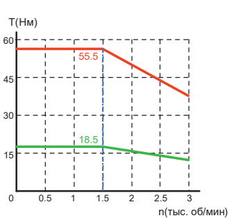
V9E-M18D-2R915
