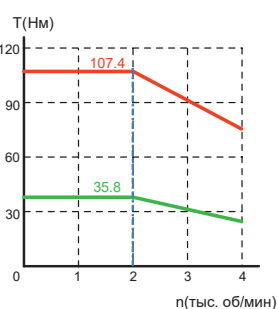
V9E-M18D-7R520
