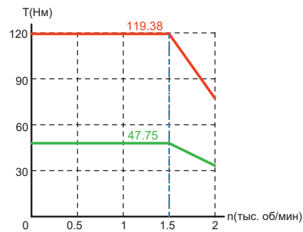
V7E-M18 □-7R515-□ □
