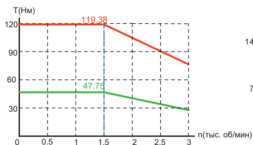
V7E-M18-7R515-□□H
