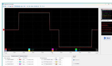
Многоканальный онлайн осциллограф для контроля в режиме реального времени (125 мкс)
