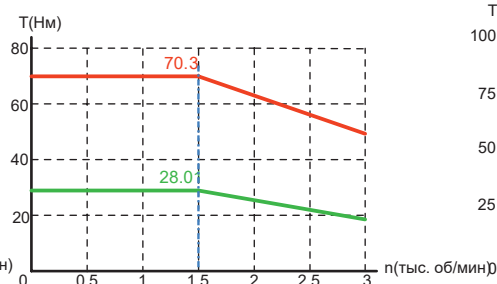
V7E-M18-4R415-□□H
