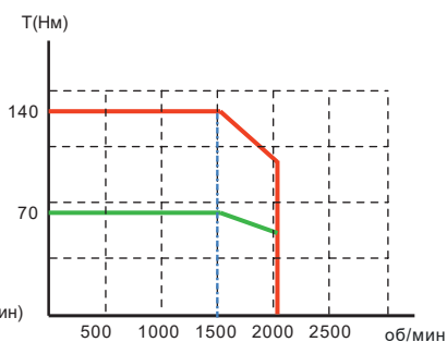
VM7-M20D-0 1115-□1FN
