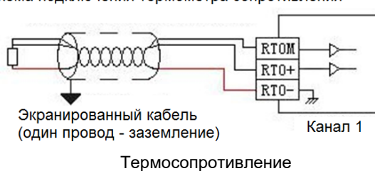
Схема подключения термометра сопротивления
