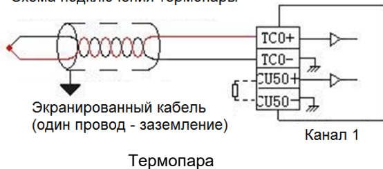
Схема подключения термопары
