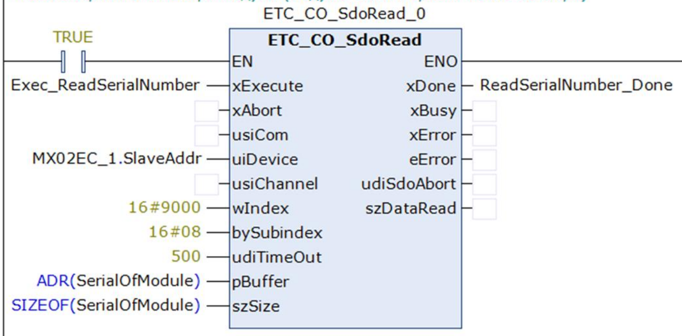
Чтение серийного номера модуля (модуль стоит первым после каплера)
