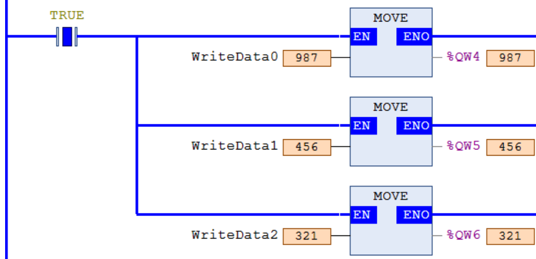
Отправка данных в регистры V3-V5 контроллера Optimus Drive AT16S0T-RU.
