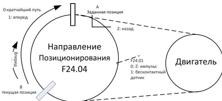
Схема направления движения при позиционировании шпинделя
