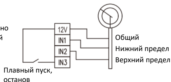
2: Контактный манометр
