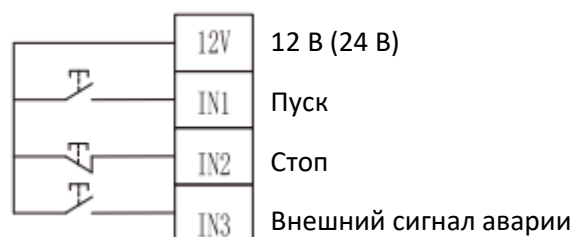
Трехпроводная система
