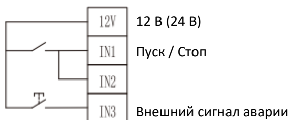
Двухпроводная система
